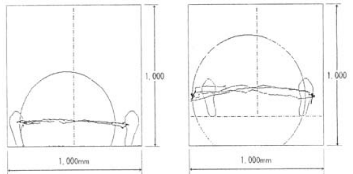
図1 スピードスケートにおけるフォームアップ時の足圧中心移動軌跡図
